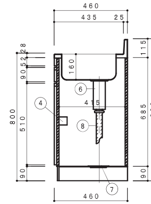
側面断面図 1/15
