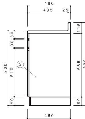
側面立面図 1/15
