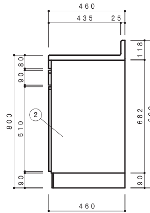
側面立面図 1/15
